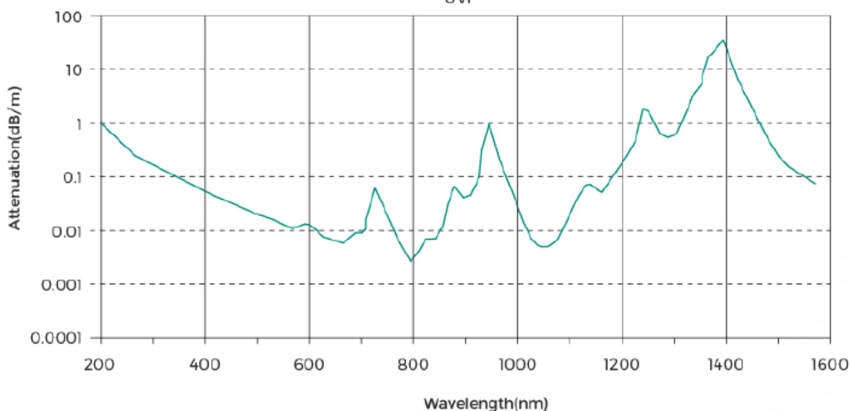
UV Attenuation Spectrum UVF
